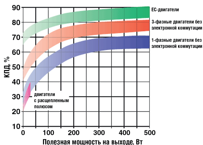
Рис. 1 Сравнение КПД двигателей различного типа
