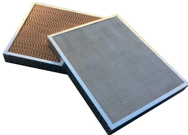
Металлическая сетка устанавливается на внешнюю часть фильтрующего блока
